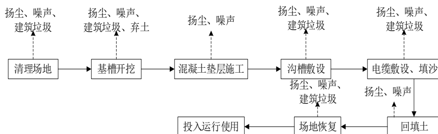
图 2-4 现状架空线路拆除施工工艺流程图
